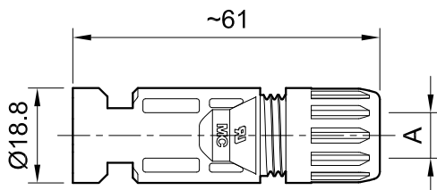
Kupplungsstecker PV-KST4...
